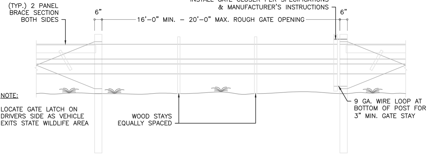
TYPICAL WIRE STRETCH GATE N.T.S.
