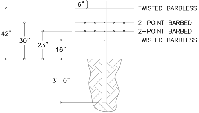
4 STRAND CATTLE FENCE N.T.S.
