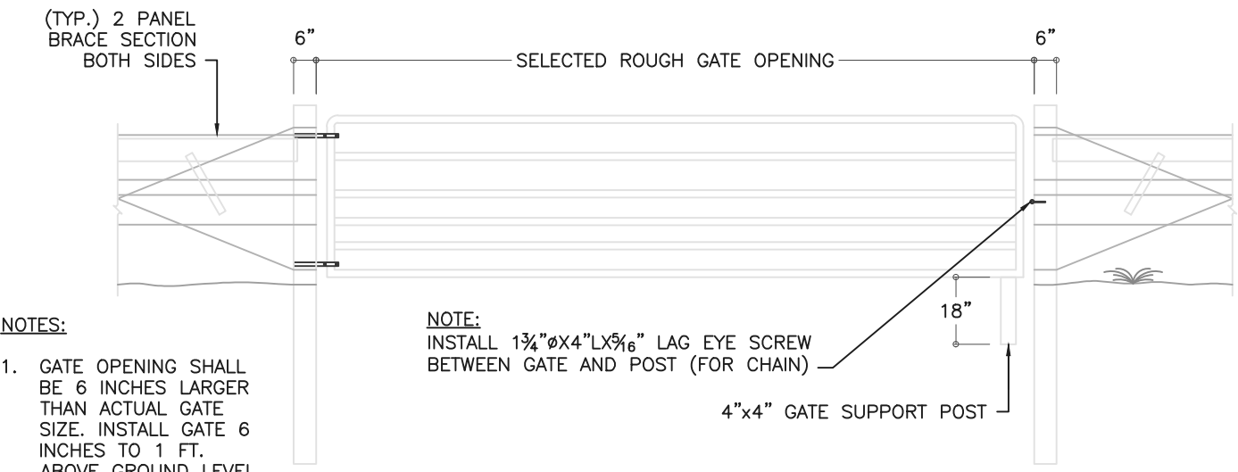
TYPICAL TUBULAR GATE N.T.S.
